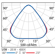
S/EW - Symmetrische extrabreite
