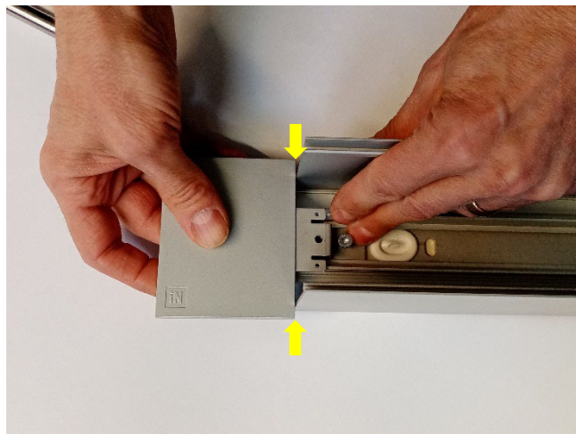
Befestigungswinkel im Kanal ausrichten Align mounting bracket in the channel
