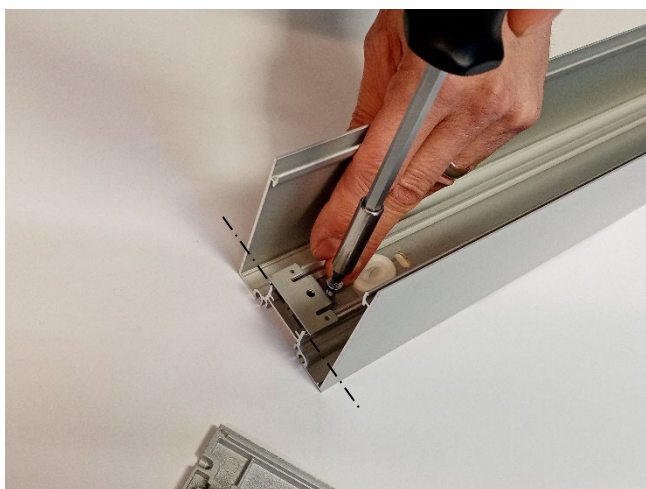
Befestigungswinkel festschrauben Screw down mounting bracket
