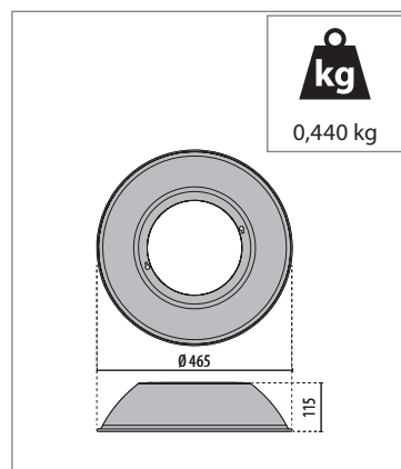
310918 - ALLUMINIUM REFLECTOR
