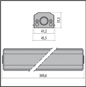
3107574 Boîtier d'alimentation DALI IN L500
