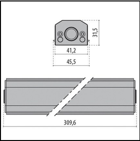
3107575 Boîtier d'alimentation DALI IN / OUT L500
