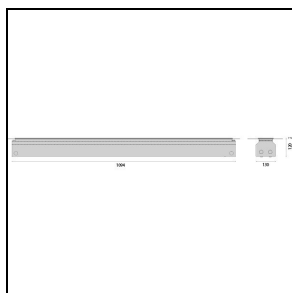
310424 Boîtier D'encastement L 1094 mm
