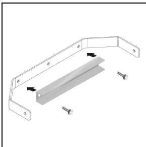
14461104 Renforcement étrier GUPELL 3. À utiliser pour fixer le projecteur avec une seule vis M10 au centre de l'étrier ■ INOX / Inox
